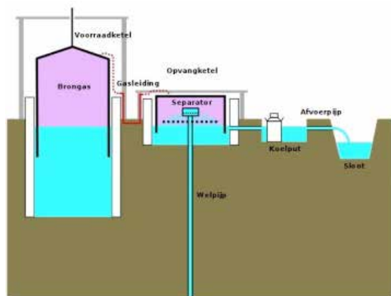
Schematische voorstelling brongaswinning
